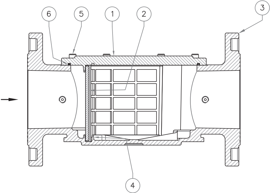
fig. 1 DN 65 - DN 80
