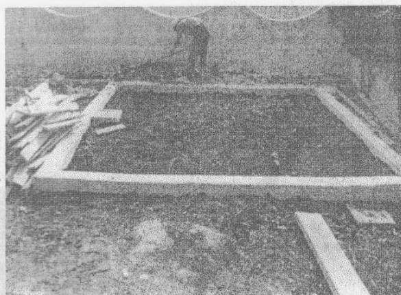
Vasoio assorbente: formazione dello strato evapotraspirante con terra vegetale e torba.
