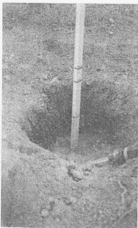
Prova di percolazione (U.S. Public Health Reprint n. 2461) per la determinazione della lunghezza della rete disperdente
