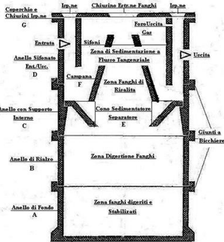
percorso dell'liquame nella fase di chiarificazione
