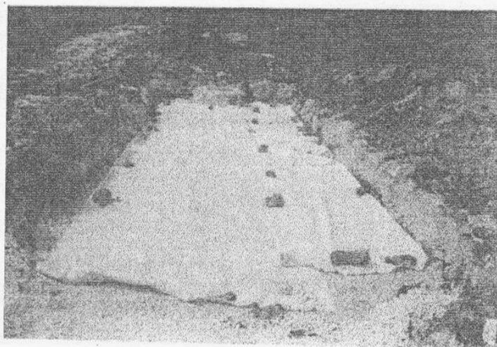
Condotta subirrigante coperta da geotessile prima del rinterro
