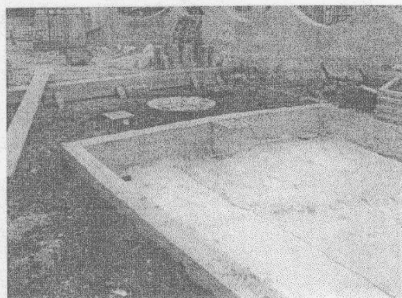
Vasoio assorbente: copertura delle condotte disperdenti con strato di geotessili
