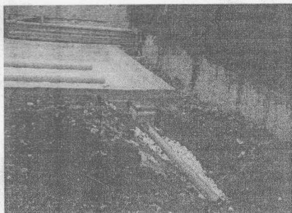
Vasoio assorbente: particolare del pozzetto di troppo-pieno e piccola condotta disperdente
