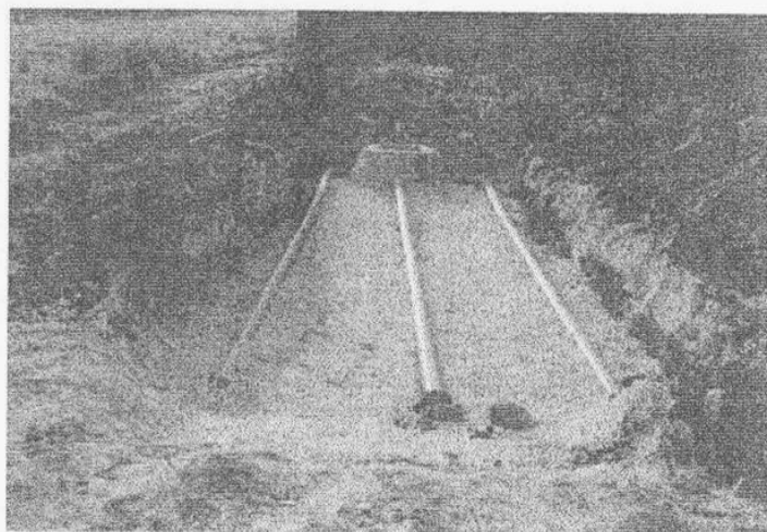
Impianto di smaltimento al suolo in trincea unica con tubi disperdenti in P.V.C. pesante disposti su tre rami paralleli
