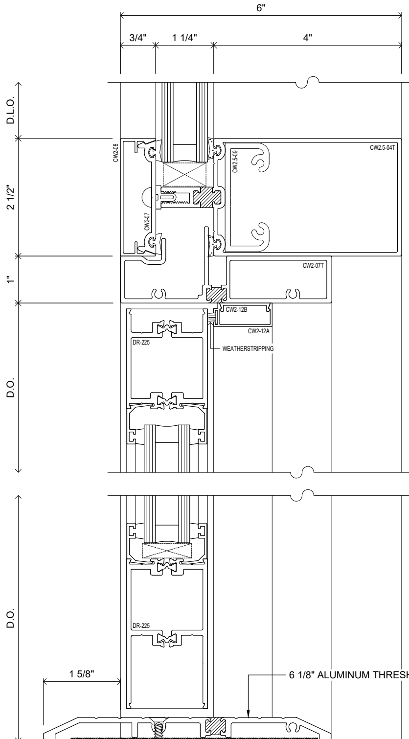
SWING DOOR HEADER DETAIL
