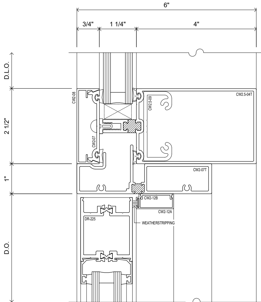
SWING DOOR HEADER DETAIL
