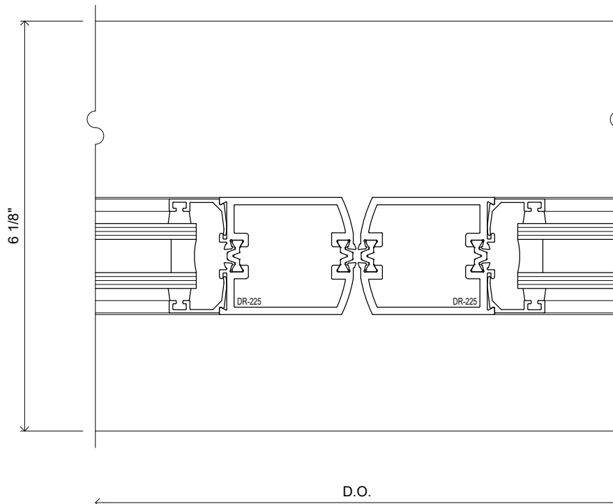
SWING DOOR JAMB DETAIL
