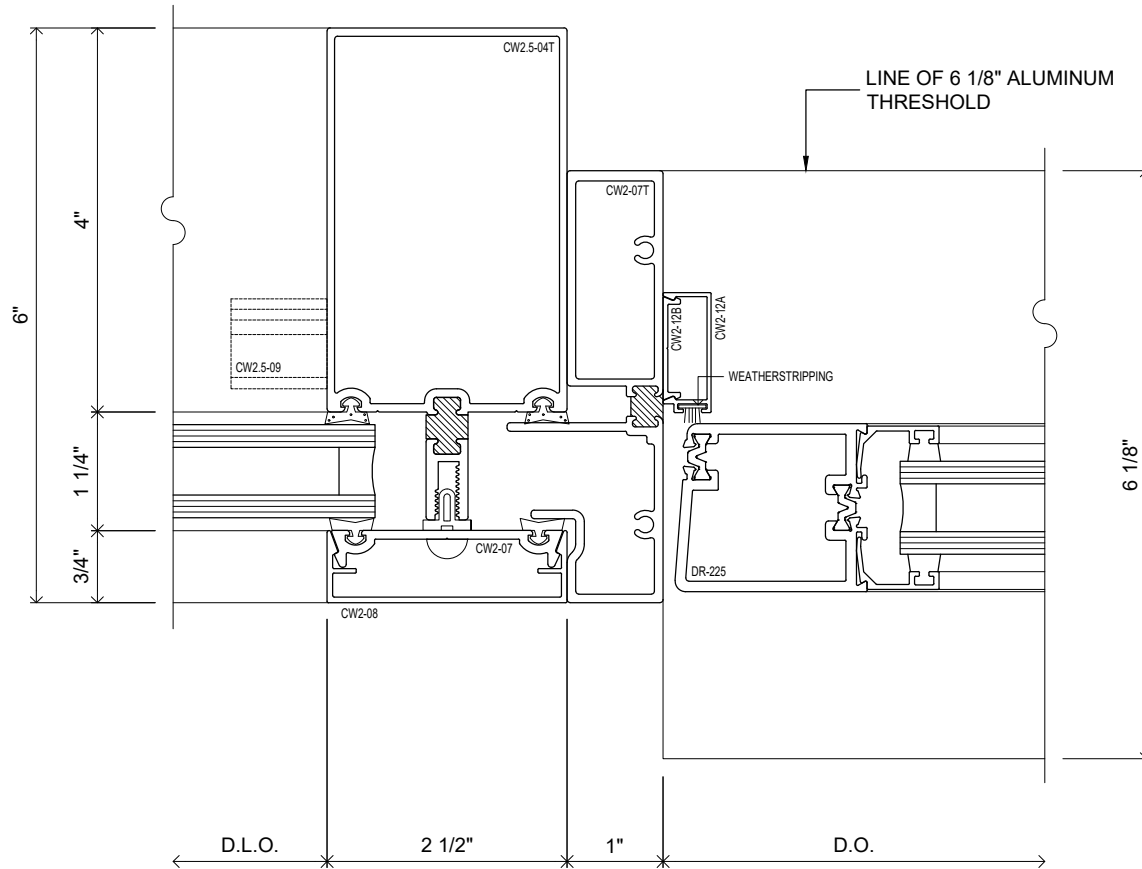
SWING DOOR JAMB DETAIL
