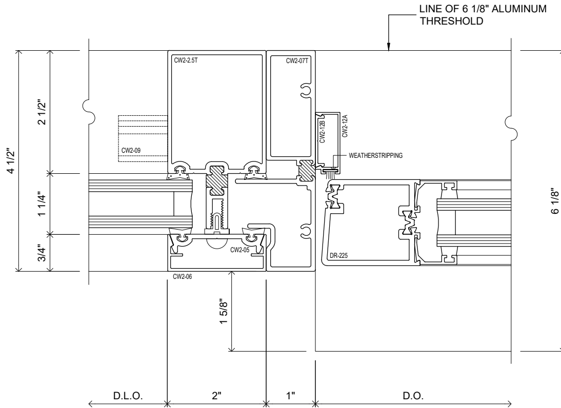
SWING DOOR JAMB DETAIL
