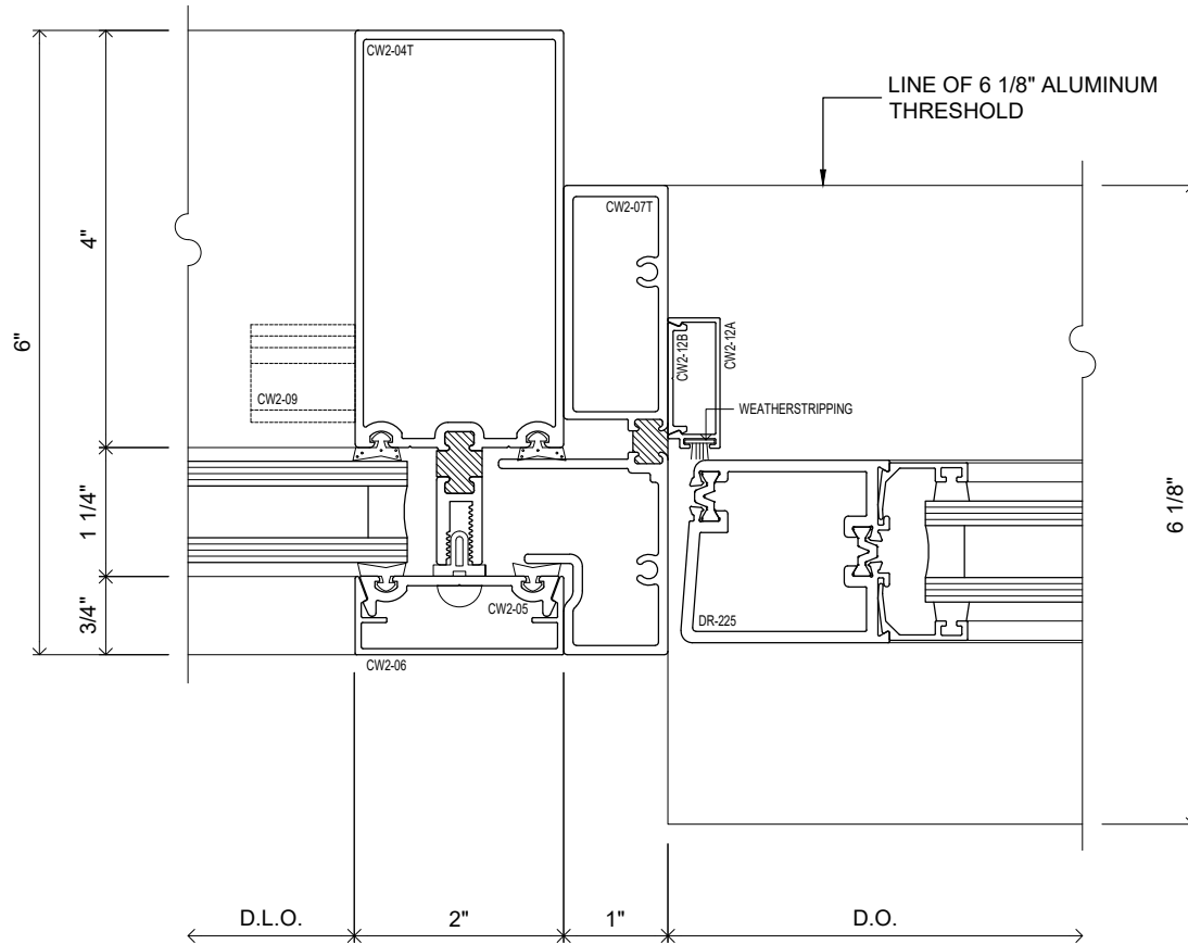
SWING DOOR JAMB DETAIL
