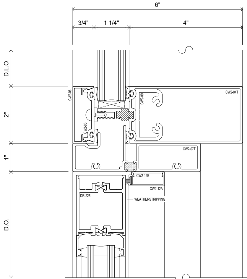
SWING DOOR HEADER DETAIL
