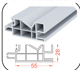
PC55 Profilo in PVC estruso da 55 mm
