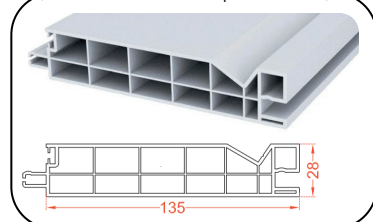
PC135 Profilo in PVC estruso da 135 mm (sostituibile con sandwich spessore 10 mm)
