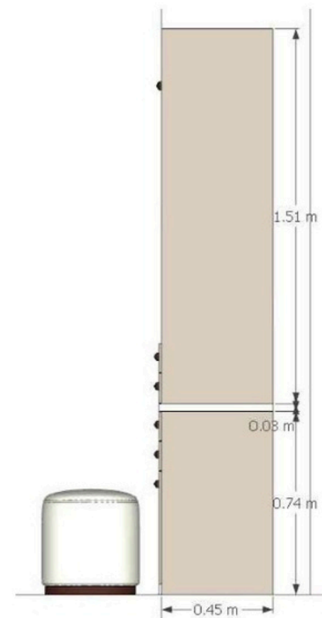
ALZADO LATERAL
