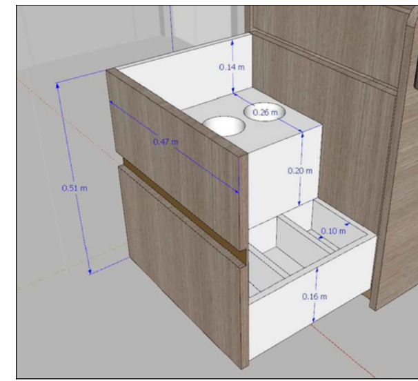
FRENTE FALSO DE 1 CAJÓN COMPLETO
