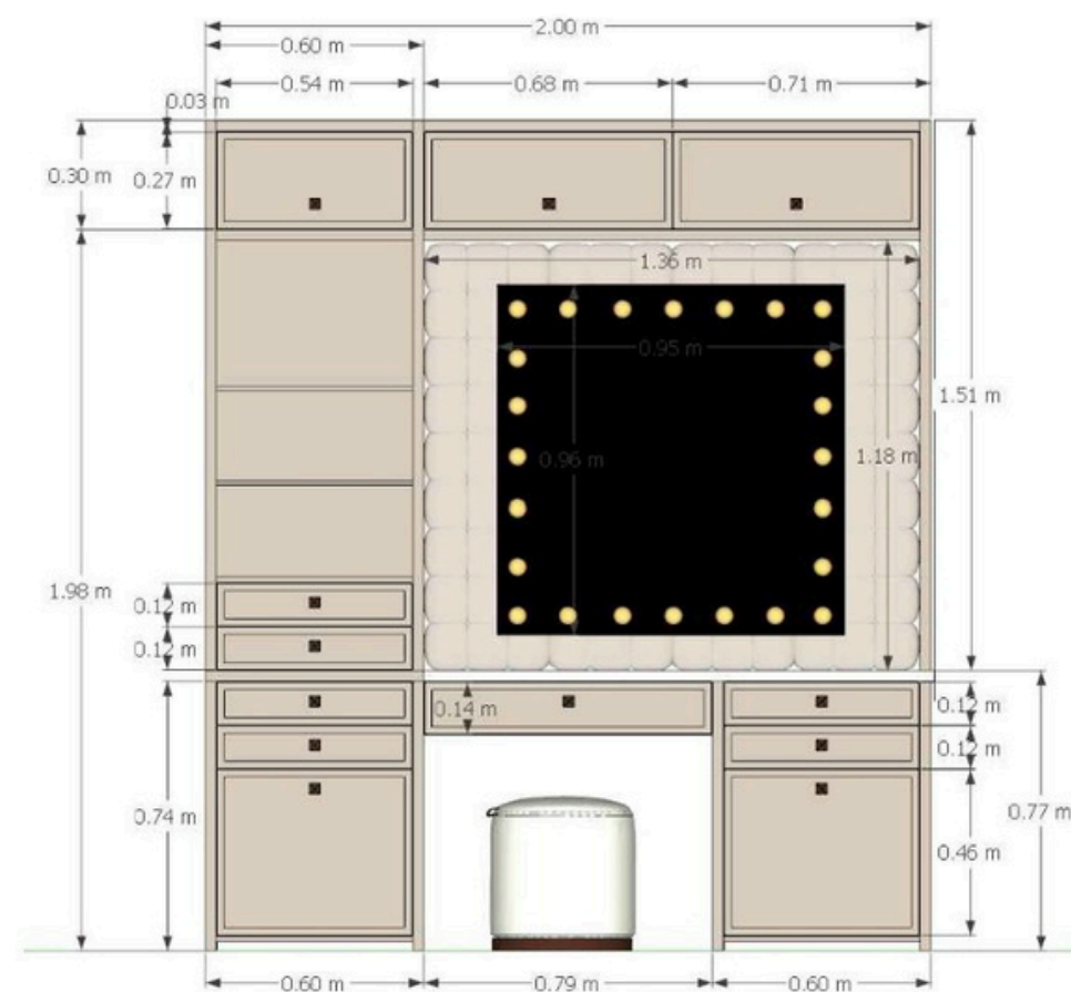
ALZADO FRONTAL DE VANITY
