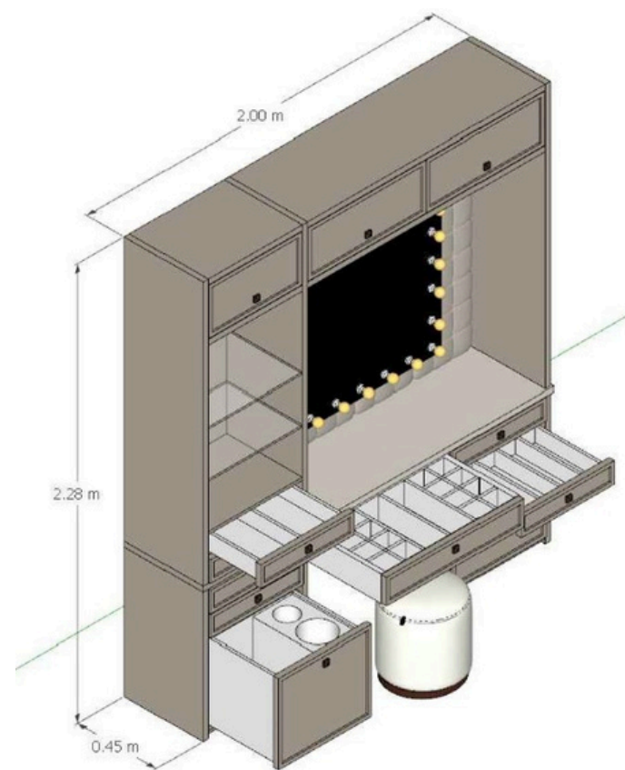
ISOMETRICO
