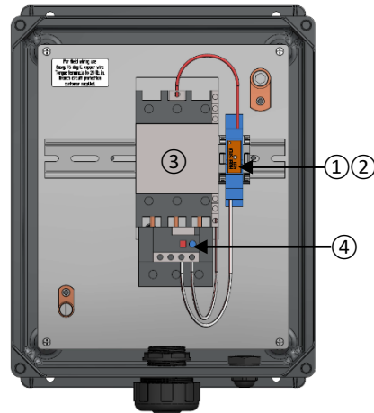
37-A. 25HP MOTOR STARTER BOX
