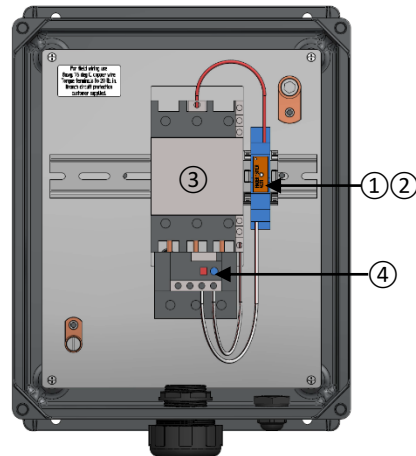
38-A. 25HP MOTOR STARTER BOX
