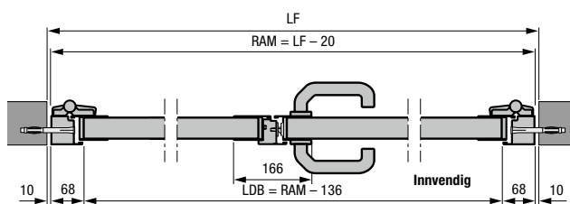
2-fløyet sidedør med blokkarm av aluminium, profiltype 2 Montering i åpningen
