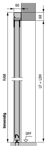
Sidedør med blokkarm av aluminium, profiltype 2 Montering bak åpningen
