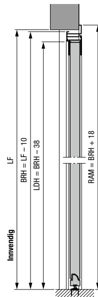
Sidedør med hjørnekarm av aluminium profiltype 2 Utvendig montering
