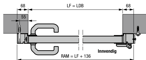
Sidedør med blokkarm av aluminium, profiltype 2 Montering bak åpningen
