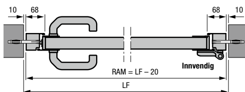
Sidedør med blokkarm av aluminium, profiltype 2 Montering i åpningen
