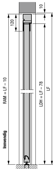
Sidedør med blokkarm av aluminium, profiltype 2 Montering i åpningen
