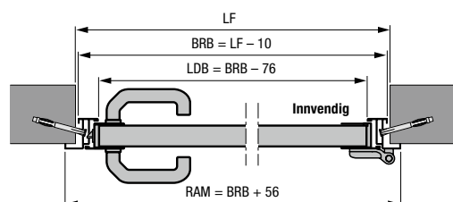
Sidedør med hjørnekarm av aluminium profiltype 2 Innvendig montering
