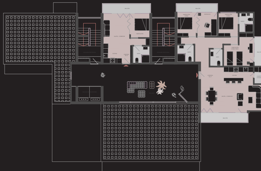
planta 13
