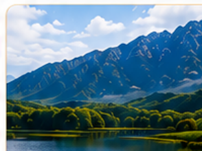
大九湖
