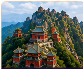
武當山金頂
