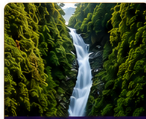
雲龍河地縫
