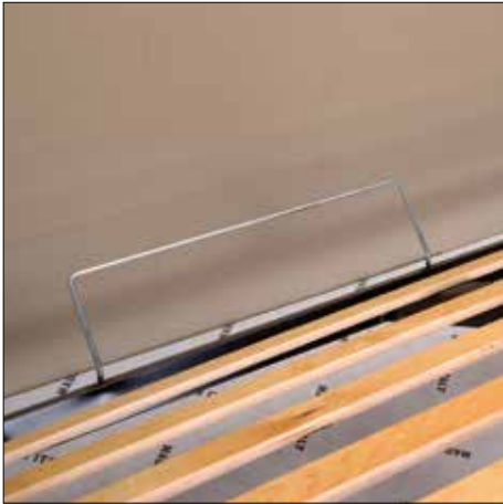
Ferma materasso
