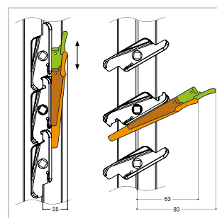
Leva premontata "BLOCK" con dispositivo di blocco e orientamento graduale delle lamelle.
