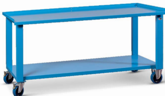
PORTATA 600 KG MM 1500 X 700 X 870H
