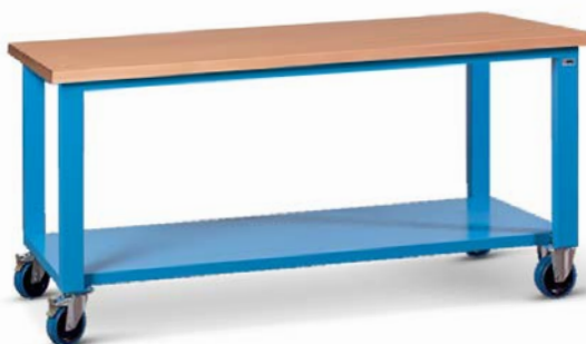
PORTATA 600 KG MM 1500 X 700 X 905H
