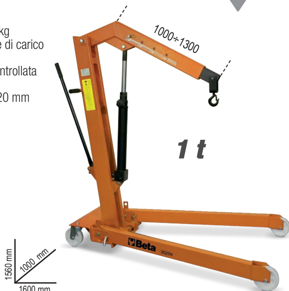
Gru idraulica pieghevole con pompa a doppio effetto
