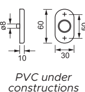
sottorosetta in plastica
