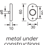
sottorosetta in metallo
