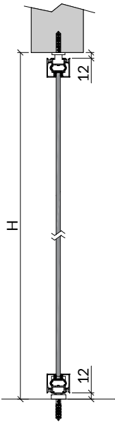
Sezione verticale muro a vista Vertical section exposed wall
