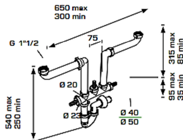
SIFONE SALVASPAZIO 2VIE C/SC.LAVATRICE (1520CP40BO)
