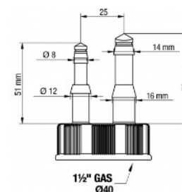
SIFONE SALVASPAZIO ISPEZIONABILE CON DOPPIO ATTACCO (A8500.01)
