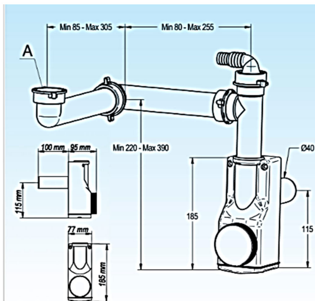
SIFONE SALVASPAZIO 1-VIA (91289.01)
