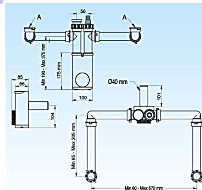
SIFONE SALVASPAZIO 2-VIE (91285.01)
