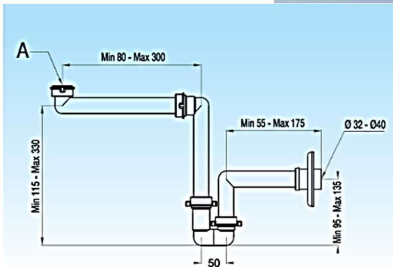
SIFONE LAVABO "SPAZIO BAGNO" (1115.01)
