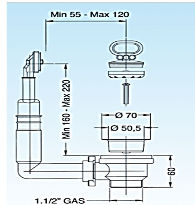
PILETTA LAVELLO "PRATICA" C/TR.PIENO (1712.000)
