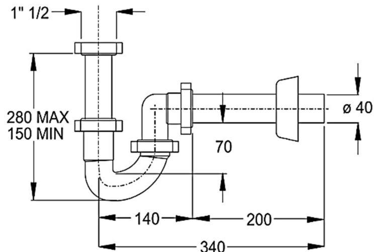
SIFONE 1VIA AUTOPULENTE (1490CP40BO)
