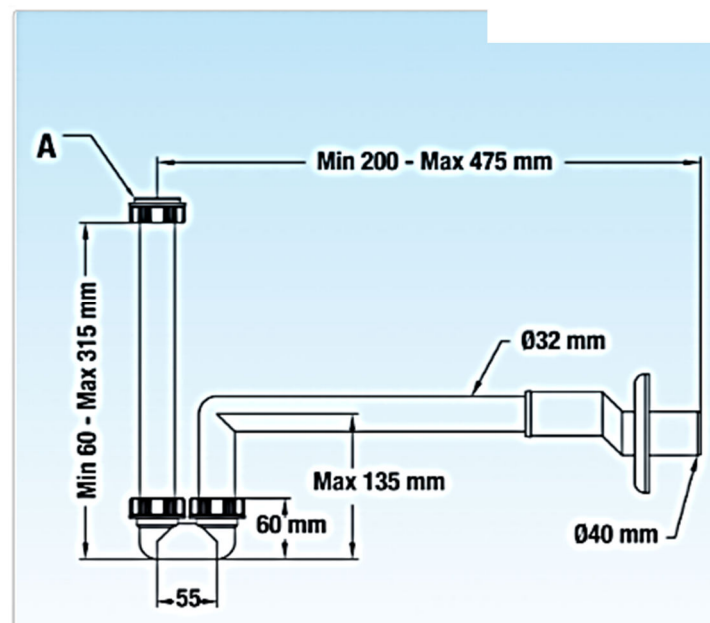
SIFONE ECCENTRICO (1643.001)
