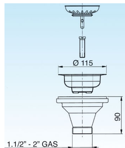
PILETTA LAVELLO "BASKET" C/GRIGLIA (1945.040)
