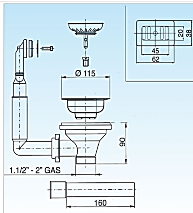
PILETTA LAVELLO "BASKET" C/TR.PIENO (1745.040/080)
