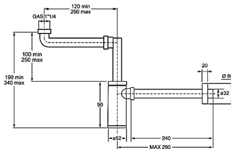
SIFONE "KING" SALVASPAZIO Ø32 (595SP25K7)
