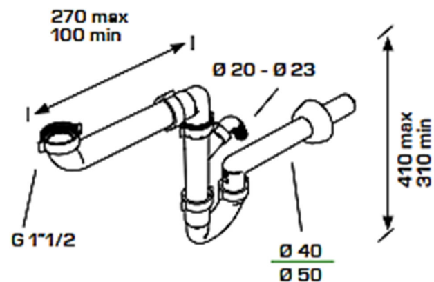
SIFONE SALVASPAZIO 1VIA C/SC.LAVATRICE (1550CP40BO)
