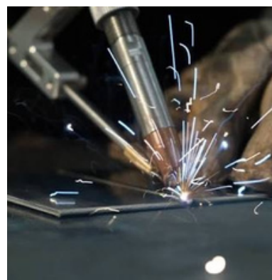
SOLDADURA LÁSER
