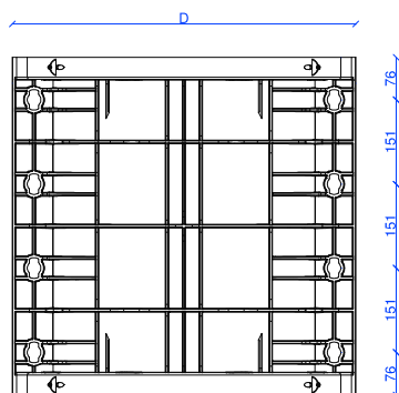
VISTA ESTERNA
