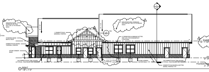
4 RIGHT 1/8" = 1'-0"
