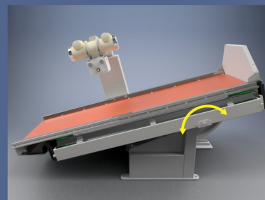
Rotación de camilla: +90°/-15°
