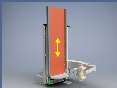
Traslación longitudinal de Camilla: 450 mm & 120 kg.
