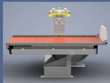
Rotación del tubo: +90°/-90° (Opcional)
