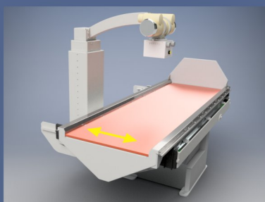
Traslación transversal de camilla: +150 mm/-150 mm
