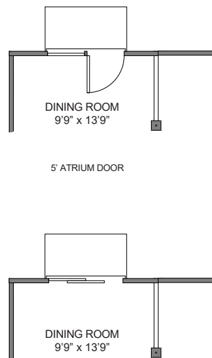
5' SLIDING DOOR
