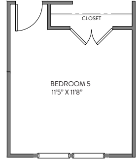
BEDROOM 5
