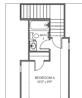
BEDROOM 4
