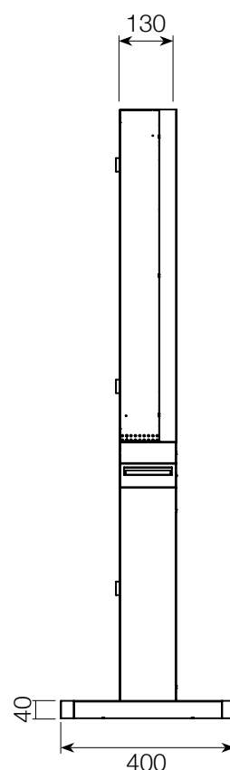
LINKE SEITE
