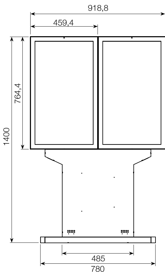
VORDERSEITE
