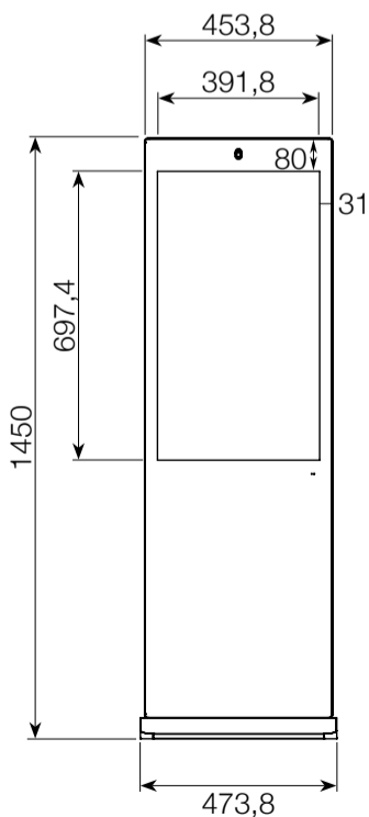
VORDERSEITE
