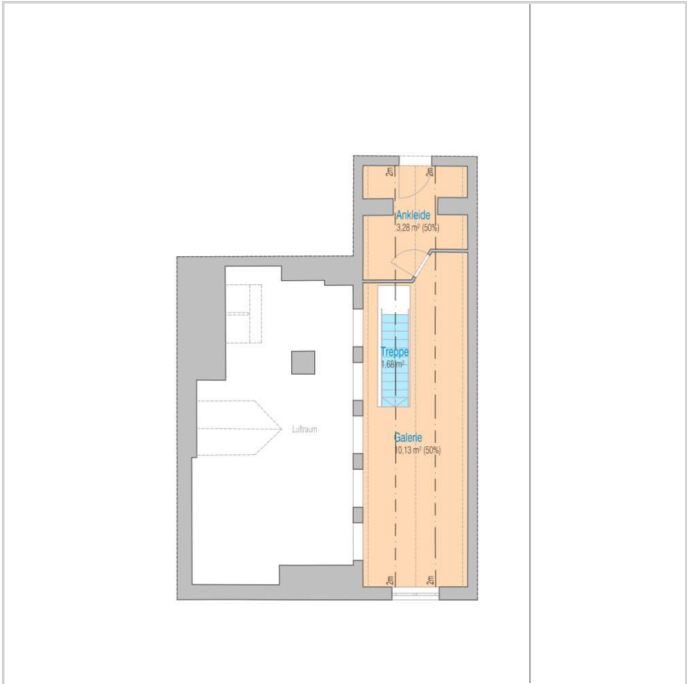
Grundriss DG
