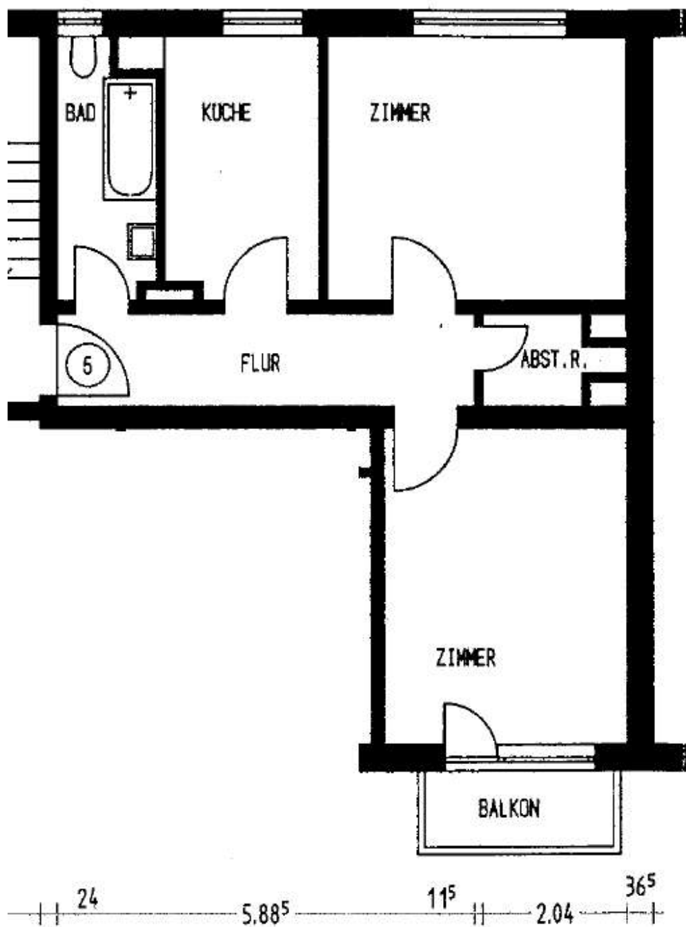
Grundriss
