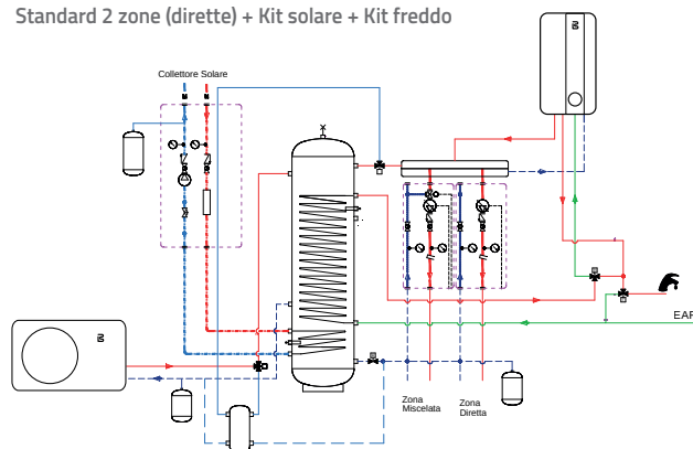
Standard 2 zone (1 diretta e 1 miscelata)
