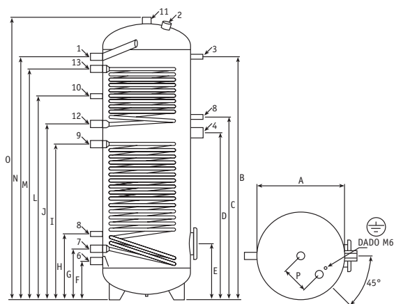
Bollitori solari da 200 a 500
