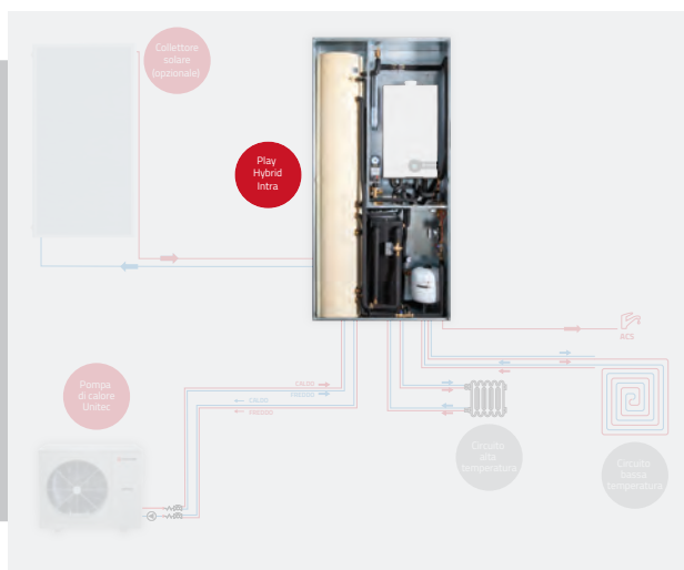
Standard 2 zone (dirette) + Kit solare + Kit freddo
