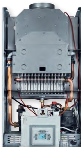
Scambiatore primario
