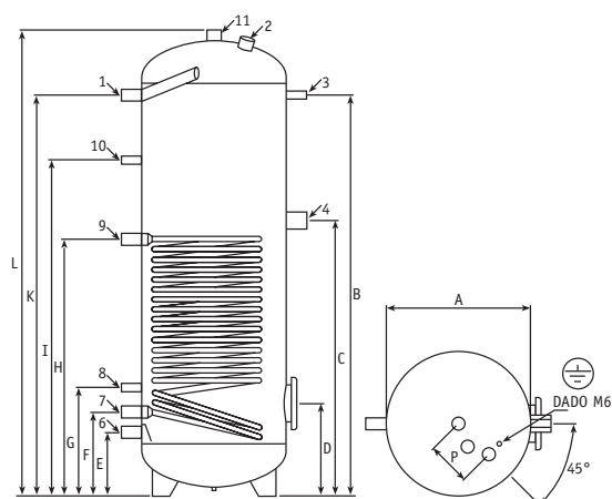
Bollitori solari da 200 a 500
