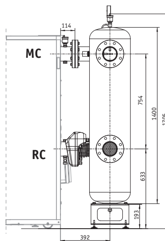
Con separatore idraulico a 90°
