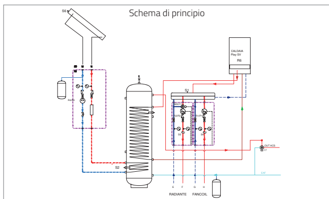
Comando remoto di serie nella versione 2 zone
