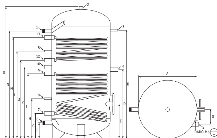
Bollitori solari da 800 a 2000
