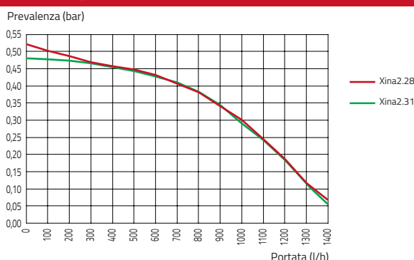
Gruppo idraulico
