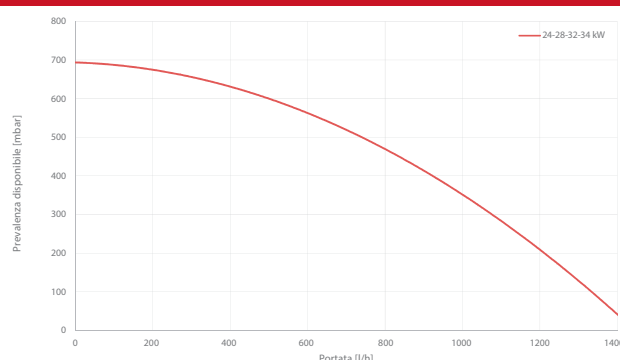
Scambiatore secondario
