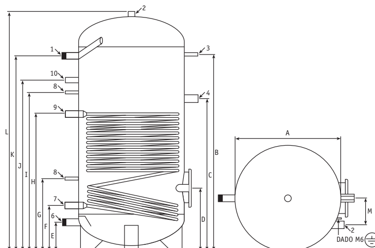
Bollitori solari da 800 a 2000
