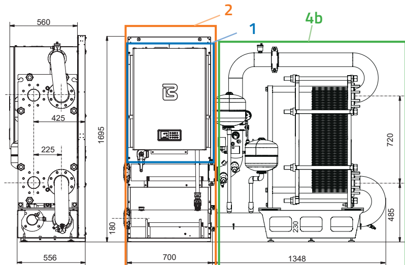
Configurazione con scambiatore a piastre >500kW
