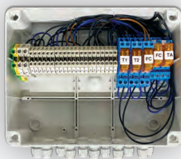
Quadro elettrico
