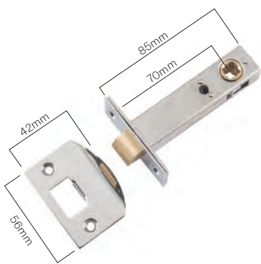
6220 PN B70mm
