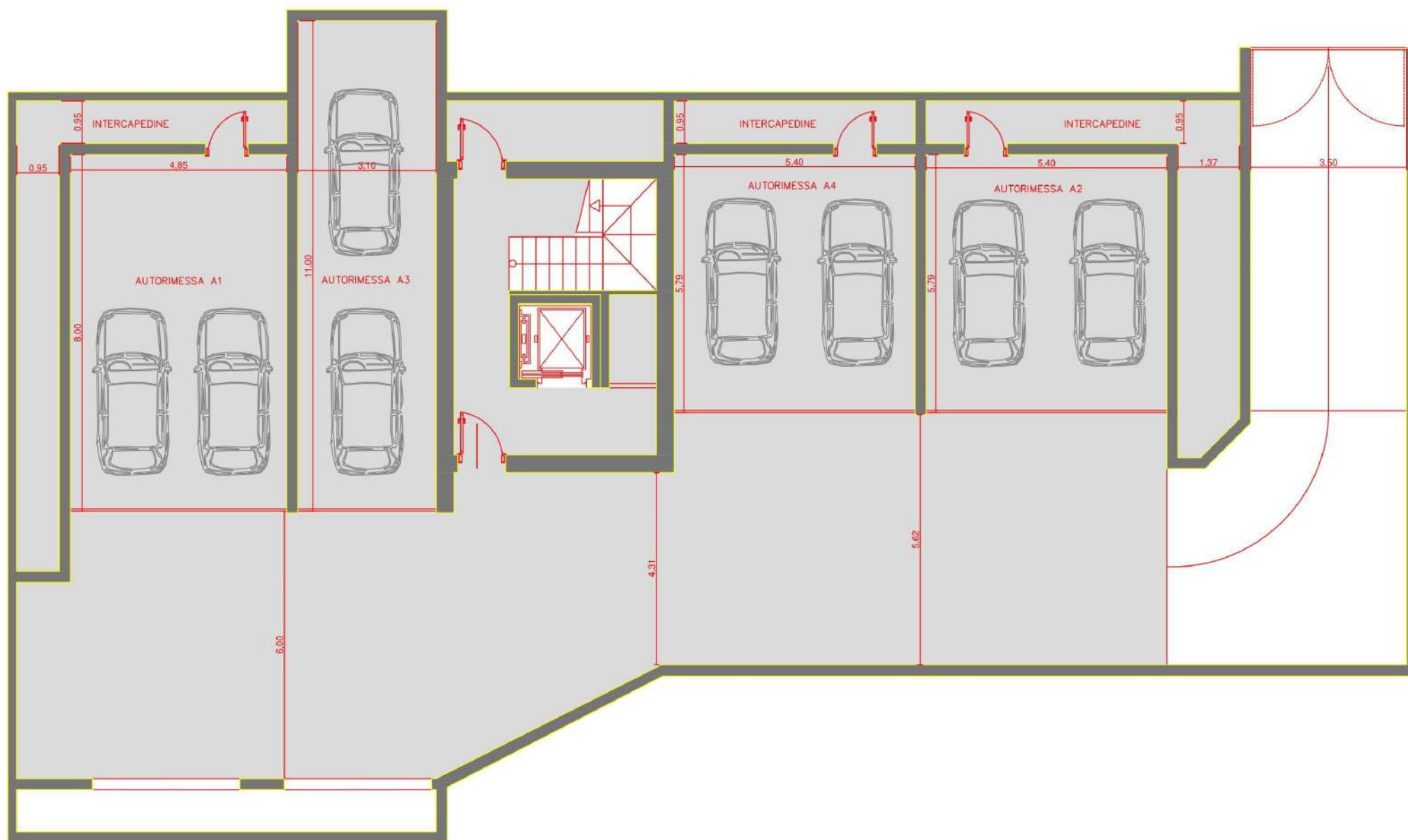
PLANIMETRIA GENERALE INTERRATO
