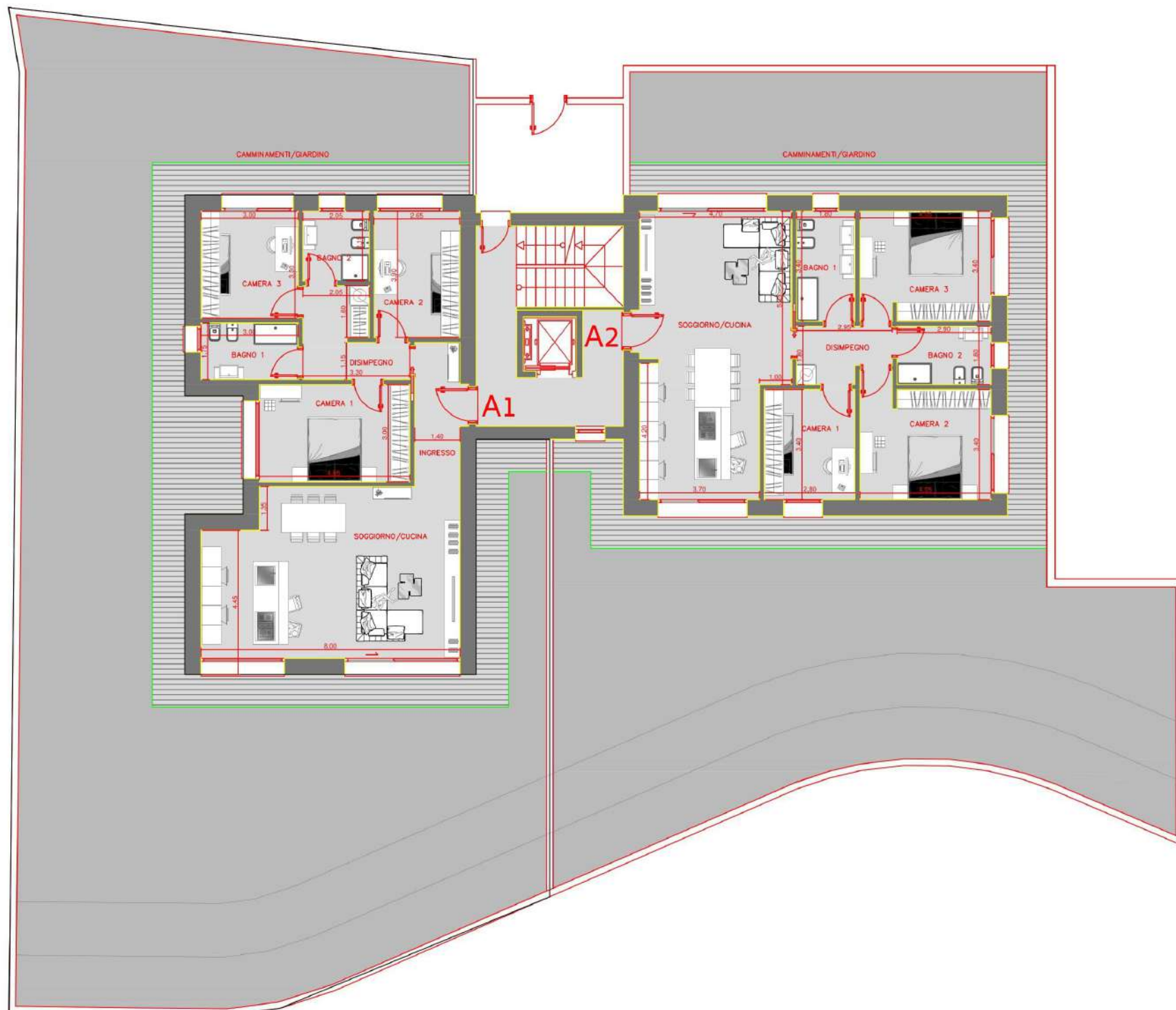
PLANIMETRIA GENERALE PIANO TERRA
