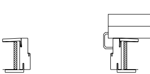
Libro-traslante _Folding-pivot NTCPKVSM
