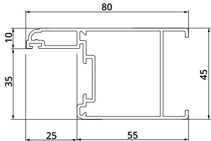
ANTA DOOR
