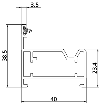
TELAIO VICENTINA VICENTINA FRAME
