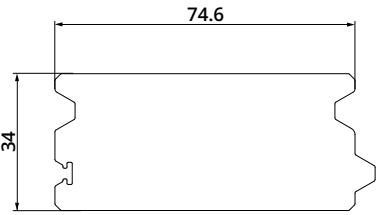
DOGA SLAT
