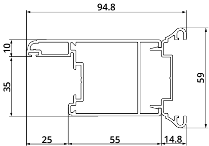
ANTA DOOR
