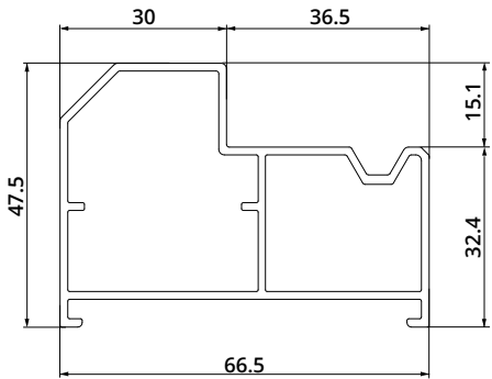
TELAIO SCURETTO SCURETTO FRAME
