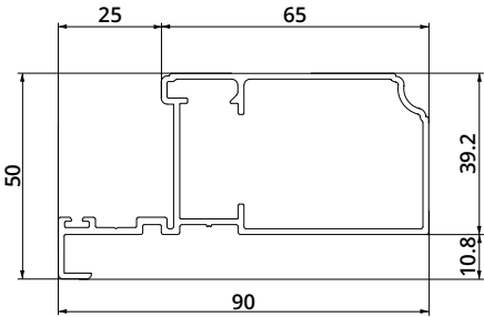
ANTA DOOR
