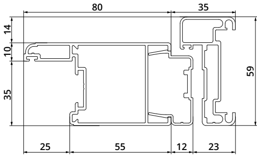
ANTA DOOR
