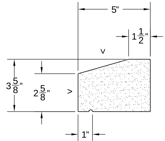
SECTION A-A SCALE 1 : 4
