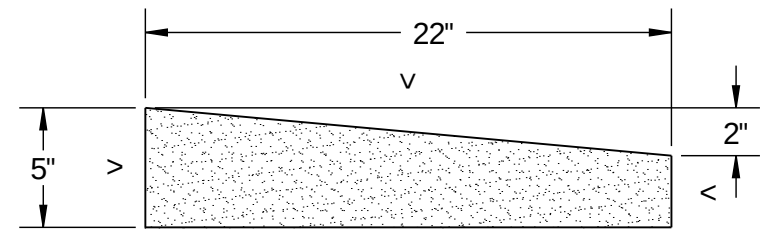
SECTION A-A SCALE 1 : 8
