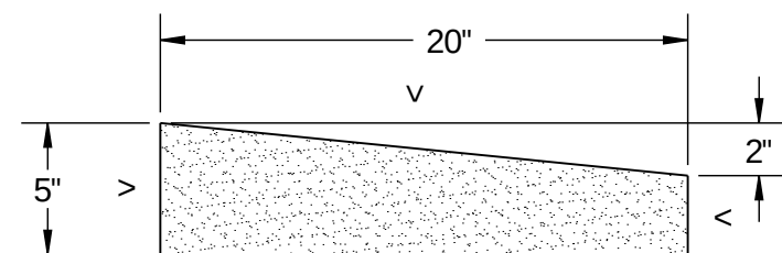
SECTION A-A SCALE 1 : 8
