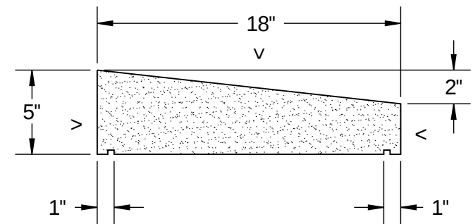
SECTION A-A SCALE 1 : 8
