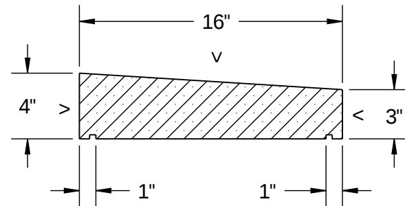
SECTION A-A SCALE 1 : 8
