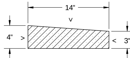
SECTION A-A SCALE 1 : 8
