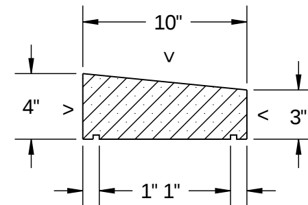
SECTION A-A SCALE 1 : 8
