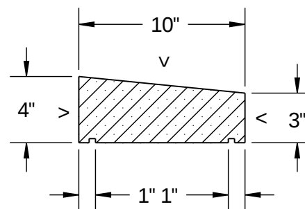
SECTION A-A SCALE 1 : 8
