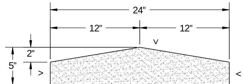
SECTION A-A SCALE 1 : 8
