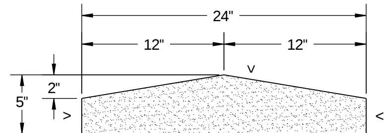
SECTION A-A SCALE 1 : 8
