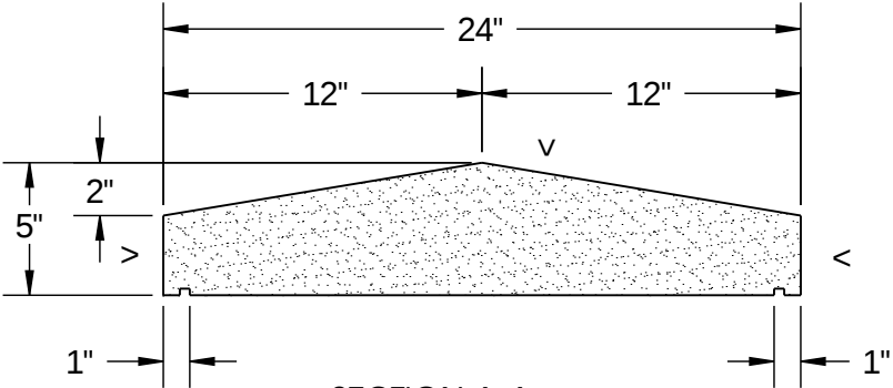
SECTION A-A SCALE 1 : 8
