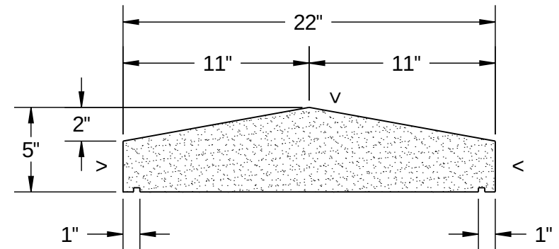
SECTION A-A SCALE 1 : 8
