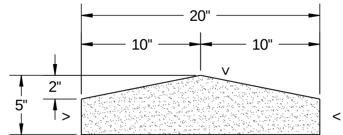
SECTION A-A SCALE 1 : 8
