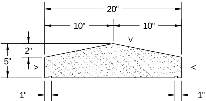
SECTION A-A SCALE 1 : 8
